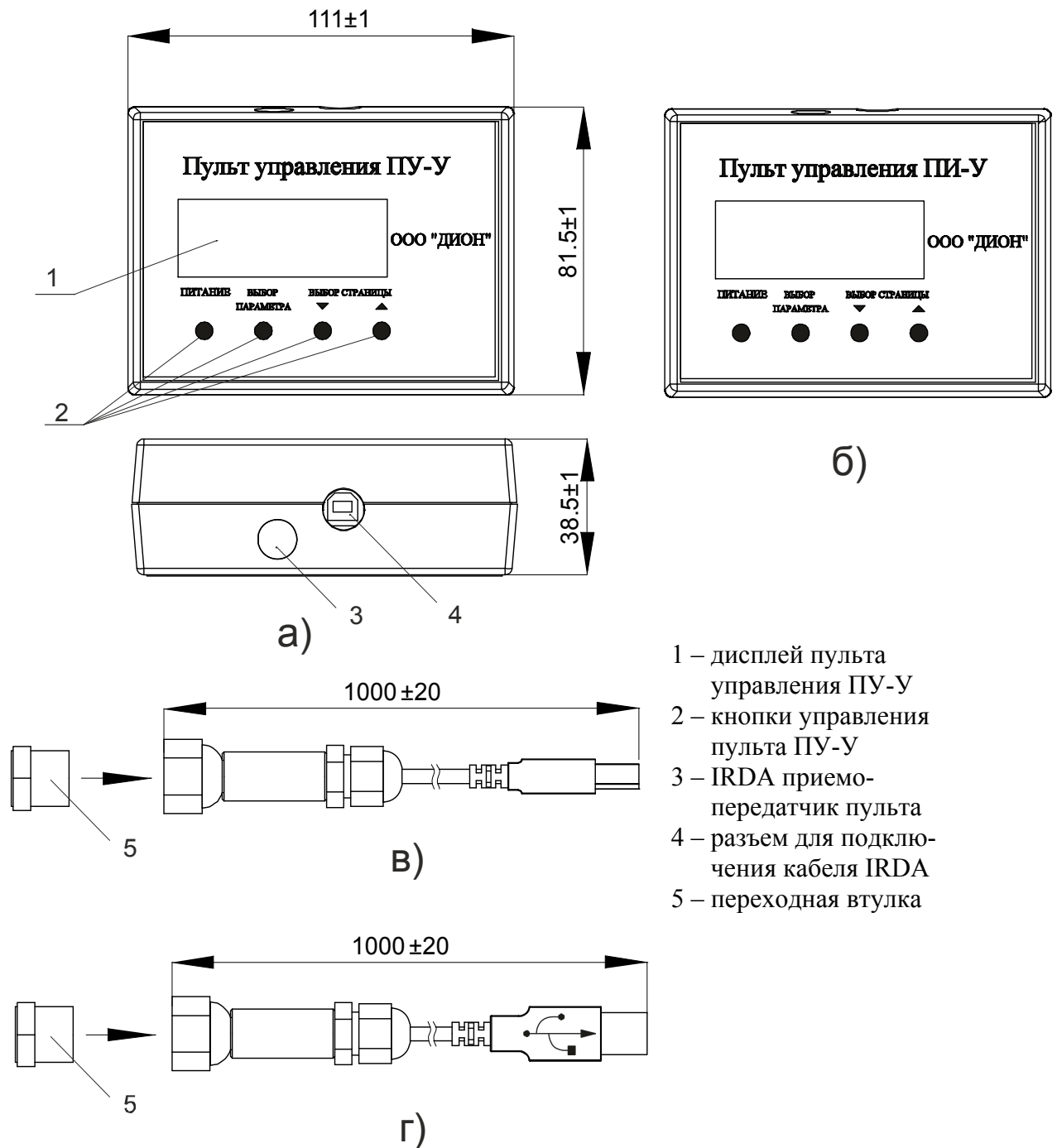
Рисунок 2. - Внешний вид и габаритные размеры пультов ПУ-У и ПИ-У, кабеля IRDA и Адаптера IRDA USB. (а – пульт управления ПУ-У; б – пульт индикации ПИ-У; в – кабель IRDA; г – Адаптер IRDA USB.)
