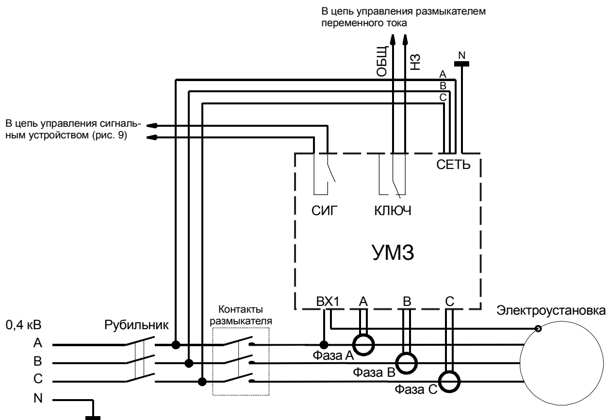
Рисунок 7. - Подключение устройства УМЗ в схему управления размыкателем переменного тока. Питание УМЗ от трех фаз.
